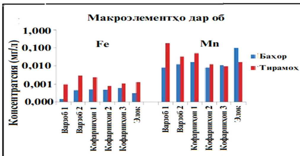
Расми 7. Тақсимшавии мавсимии элементҳо дар оби дарёҳо.
