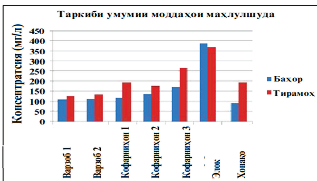
Расми 2. Тағйироти мавсимии тақсимоти таркиби умумии моддаҳои маҳлулшуда дар оби дарёҳо.
