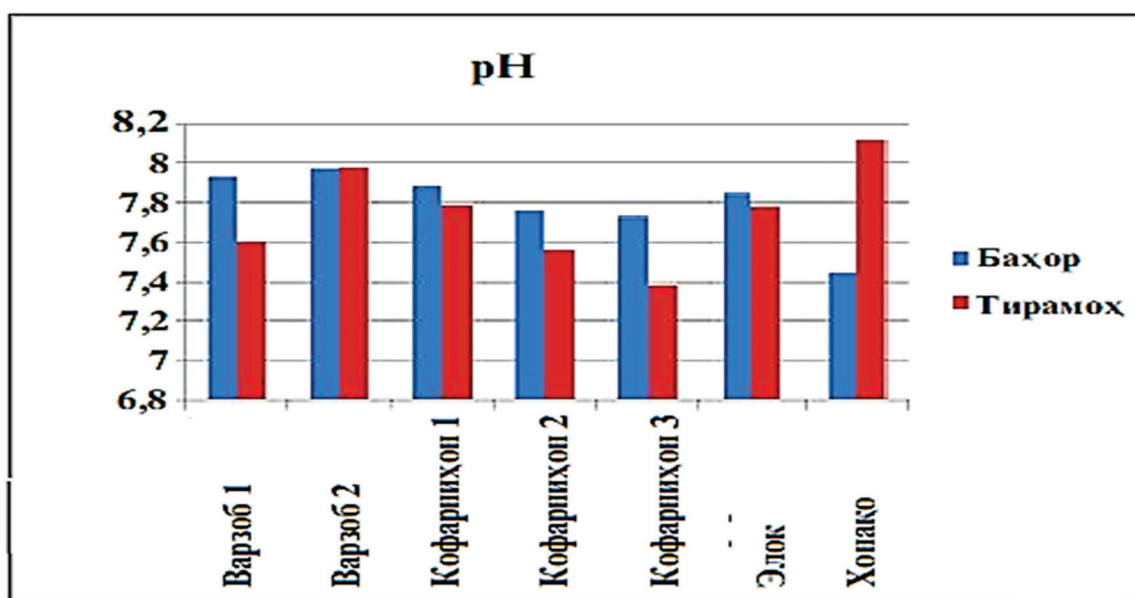
Расми 5. Тағйирёбии мавсимии қимати рН дар оби дарёҳо.
